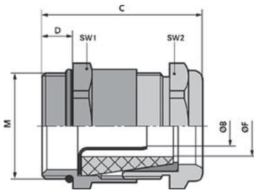
SKINDICHT® SHVE-M ATEX
